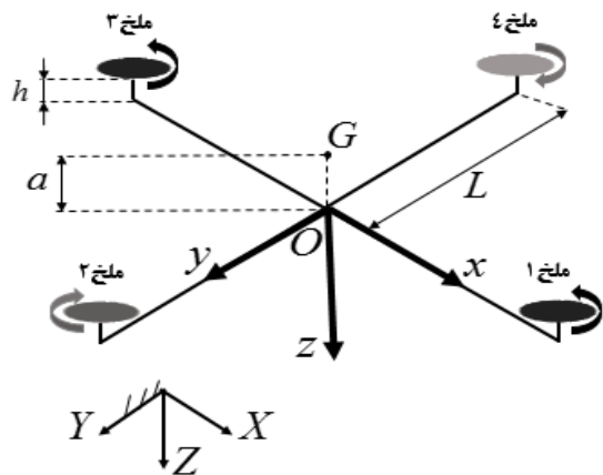
شکل ۱. نمایی از ربات چهارملخه و دستگاه‌های مختصات اینرسی و بدنی
