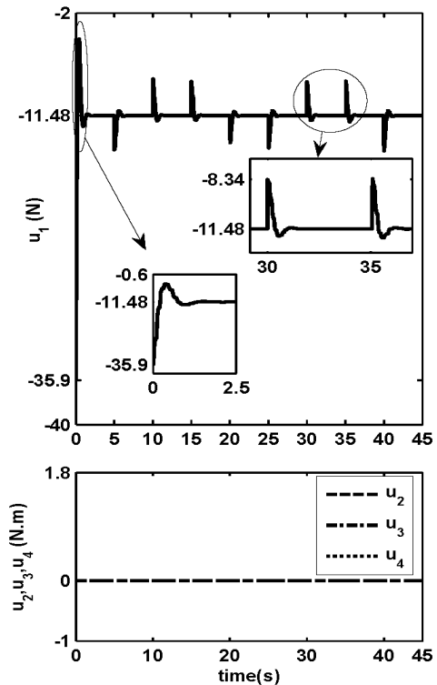
شکل ۴. ورودی‌های کنترلر
