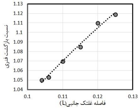
شکل ۶. نمودار تغییرات نسبت بازگشت فیزی با فاصله غلتک جانبی
