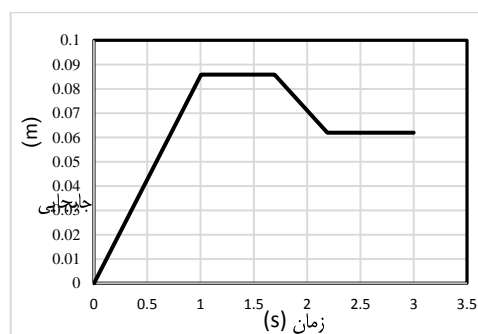
شکل ۹. الگوی جابه‌جایی غلتک جانبی در راستای افقی برحسب زمان
