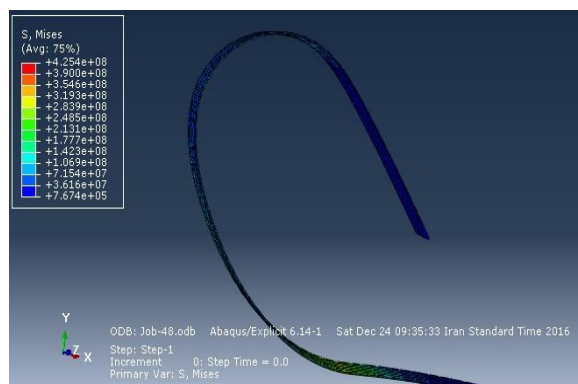
شکل ۱۱. پوسته با دو انحنای متفاوت قبل از بازگشت فتری
