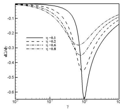
شکل ۷. حساسیت نسبت فرکانسی به نسبت کامپلینس برای فواصل مختلف از پمپ ( \lambda=0 )
