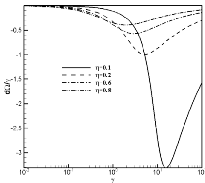
شکل ۸. حساسیت نسبت فرکانسی به نسبت کامپلینس برای فواصل مختلف از پمپ ( \lambda=1 )
