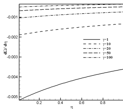
شکل ۹. حساسیت فرکانس سیستم به قرارگیری آکمولاتور برای نسبت کامپلینس متفاوت ( \lambda=0 )
