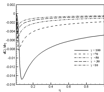
شکل ۱۰. حساسیت فرکانس سیستم به محل قرارگیری آکمولاتور برای نسبت کامپلینس متفاوت ( \lambda=1 )
