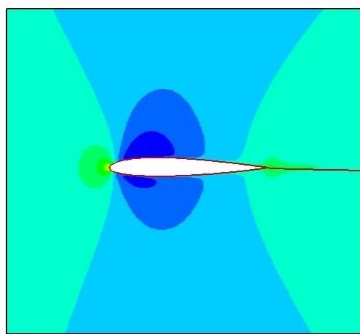
شکل ۱۲. خطوط همتراز درجه حرارت برای جریان تراکم‌پذیر غیرلزج در عدد ماخ ۰/۷ و زاویه حمله ۲ درجه
