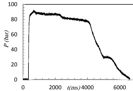
شکل ۱۱. منحنی تغییرات فشار موتور (تست موتور)
