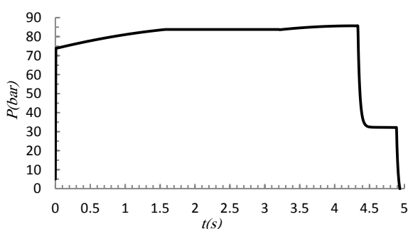
شکل ۶. تغییرات فشار در موتور
