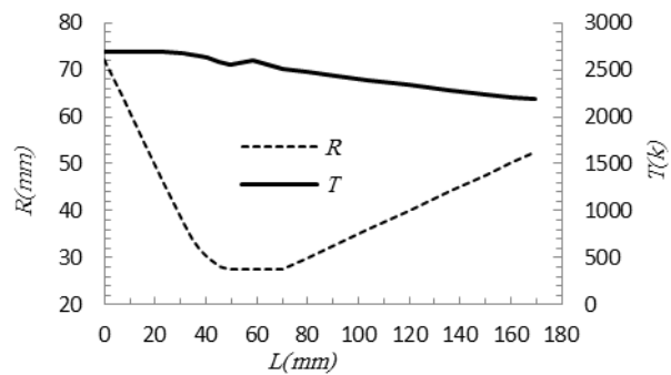
شکل ۷. تغییرات دمای دیواره در طول نازل
