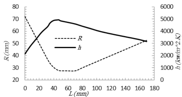
شکل ۹. منحنی تغییرات ضریب انتقال حرارت در دیواره نازل
