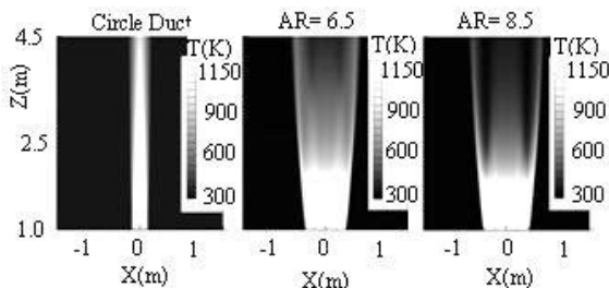
شکل ۱۹. مقایسه توزیع دما داکت با نسبت منظری ۶/۵، ۸/۵ و دایروی (XZ)
