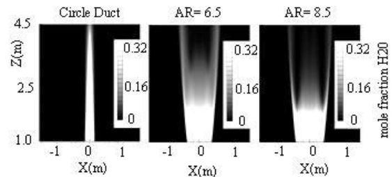
شکل ۱۷. مقایسه توزیع کسر مولی داکت با نسبت منظری ۶/۵، ۸/۵ و دایروی (XZ)
