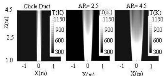
شکل ۱۸. مقایسه توزیع دما داکت با نسبت منظری ۲/۵، ۴/۵ و دایروی (XZ)
