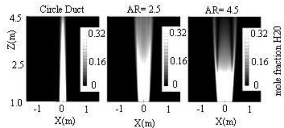
شکل ۱۶. مقایسه توزیع کسر مولی داکت با نسبت منظری ۲/۵، ۴/۵ و دایروی (XZ)
