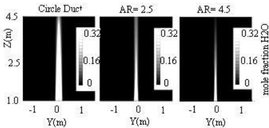
شکل ۲۰. مقایسه توزیع کسر مولی داکت با نسبت منظری ۲/۵، ۴/۵ و دایروی (YZ)
